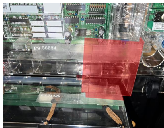
取付け位置
